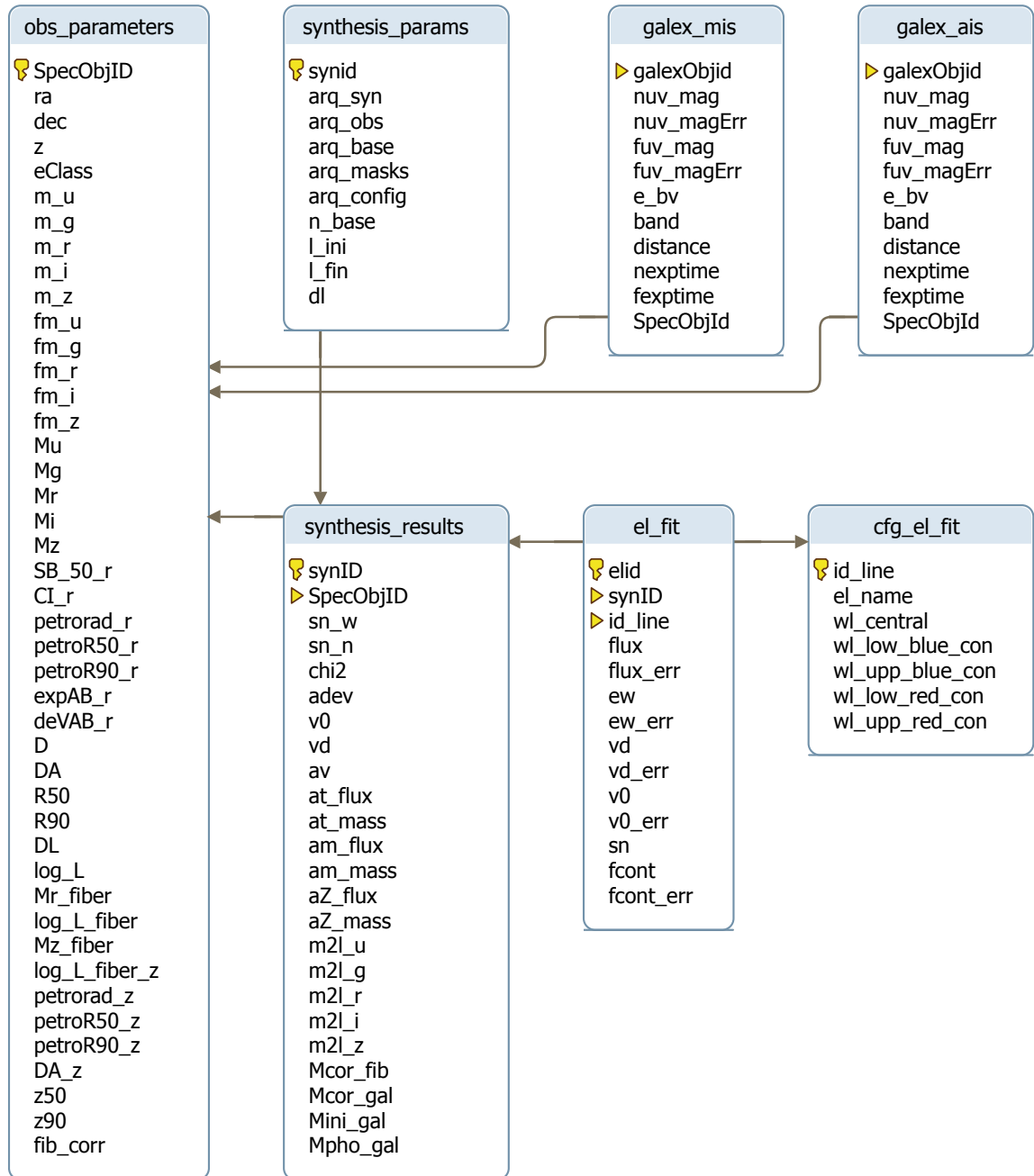
Figura 3.3: Esquema do banco de dados do STARLIGHT. As linhas indicam chaves estrangeiras, relacionando dois campos de duas tabelas diferentes.
