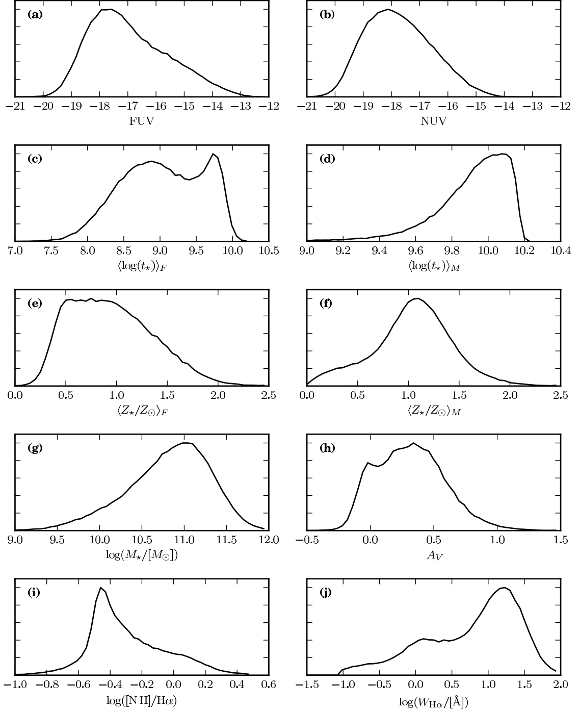
Figura 3.5: Histogramas das medidas da amostra STARLIGHT+UV .
