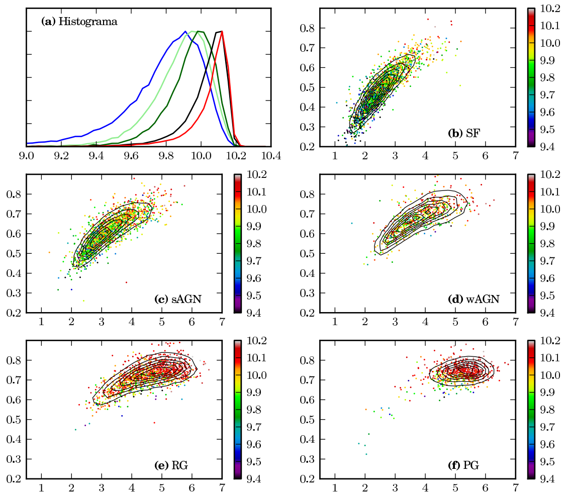
Figura 4.9: O mesmo que a figura 4.8, para a idade estelar média das galáxias, ponderada pela massa. Note que a escala de idades não é a mesma.
