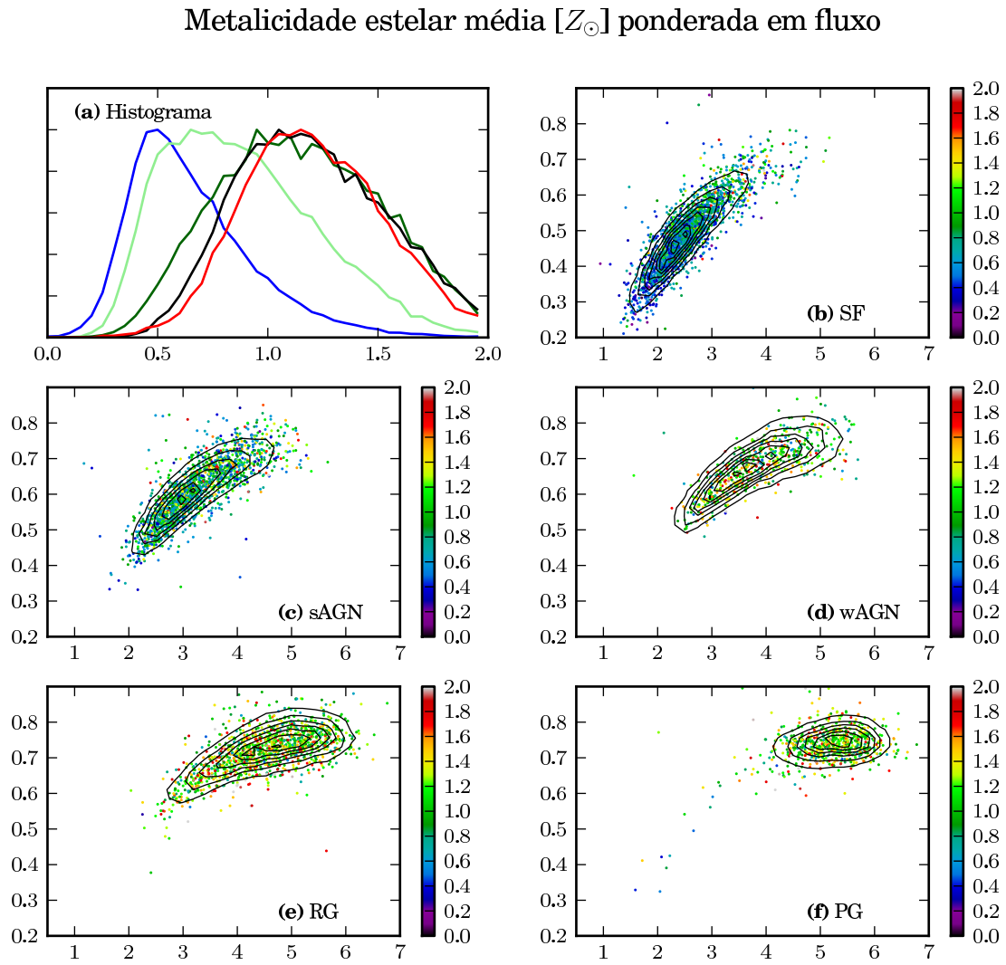
Figura 4.10: O mesmo que a figura 4.8, para a metalicidade estelar média das galáxias, ponderada pelo fluxo.
