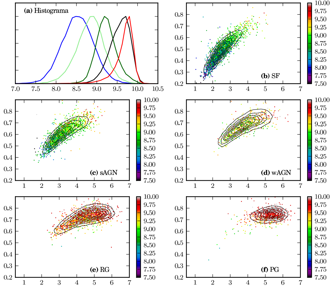
Figura 4.8: Idade estelar média das galáxias, ponderada pelo fluxo, em função de \text{NUV} - r e g - r . O painel (a) mostra o histograma normalizado das idades para cada classe, utilizando o mesmo código de cores da figura 4.3. Os painéis de (b) a (f) são diagramas cor–cor com eixos iguais aos da figura 4.1 contendo somente as galáxias com formação estelar (SF), AGN fortes (sAGN), AGN fracas (wAGN), galáxias aposentadas (RG) e galáxias passivas (PG), respectivamente. Os contornos indicam a densidade de galáxias.
