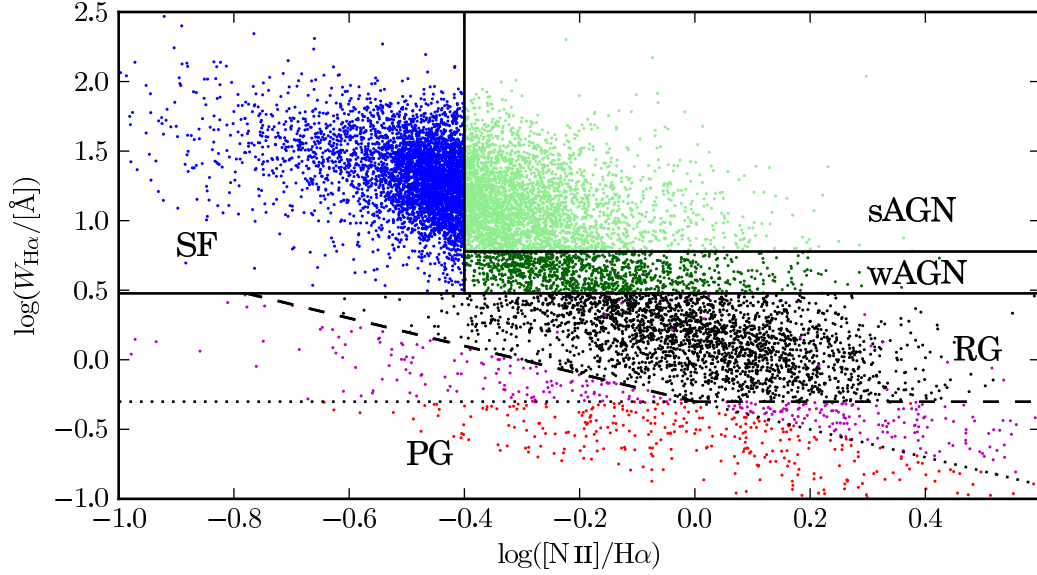
Figura 4.3: Diagrama de diagnóstico WHAN. As linhas tracejadas separam as galáxias em classes. Azul: galáxias com formação estelar (SF). Verde claro: galáxias com núcleo ativo forte (sAGN). Verde forte: galáxias com núcleo ativo fraco (wAGN). Preto: galáxias aposentadas (RG). Vermelho: galáxias passivas (PG). Magenta: Galáxias que não se encaixam em nenhuma destas classes.
