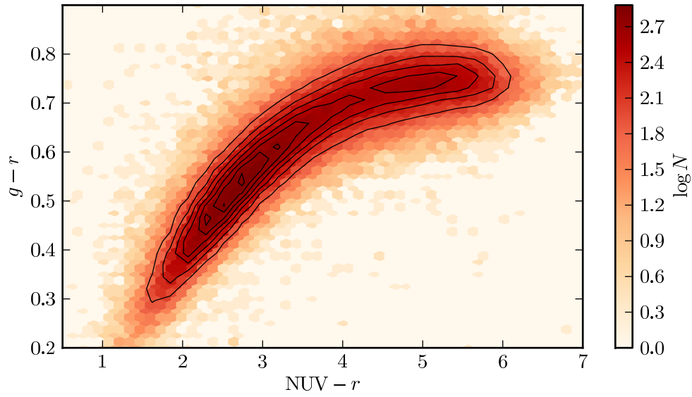
Figura 4.1: Frequência de galáxias no diagrama cor-cor ( \text{NUV} - r versus g - r ) da amostra STARLIGHT+UV.
