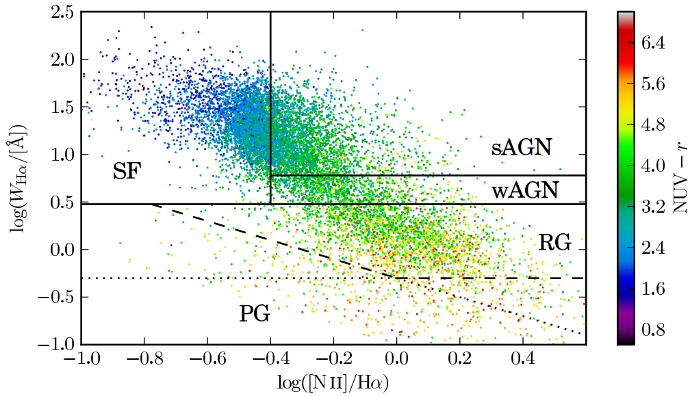
Figura 4.4: Diagrama WHAN semelhante ao da figura 4.3. A cor dos pontos representa NUV - r . Pode-se notar que a cor UV das galáxias é diferente para cada classe.
