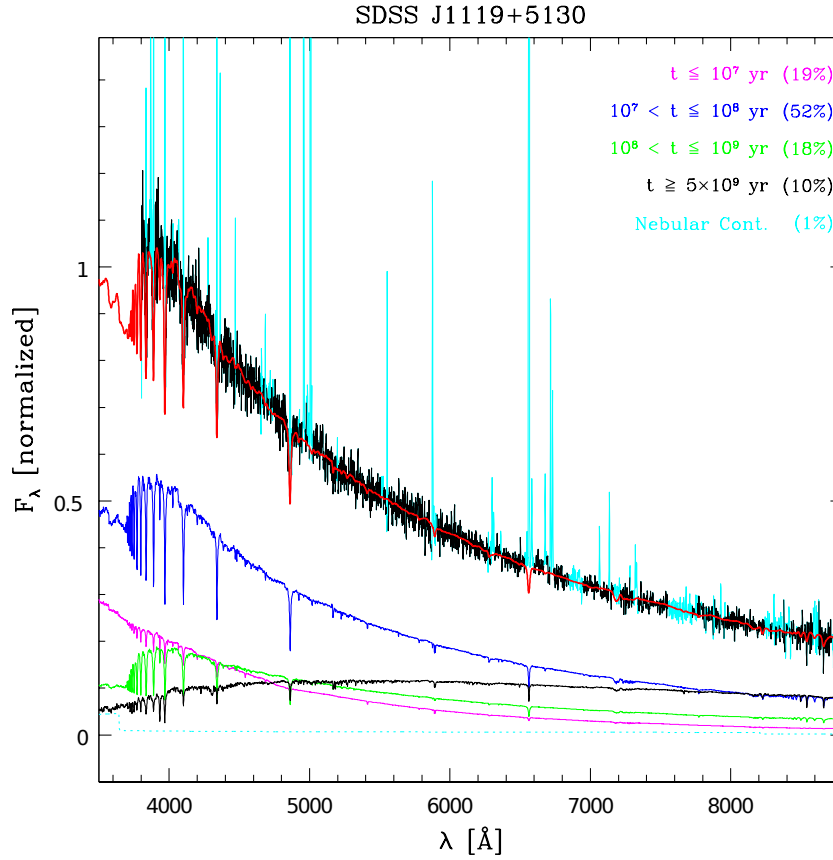
Figura 1.1: Exemplo de ajuste com o STARLIGHT para o espectro de SDSS J1119+5130 (Cid Fernandes 2006, figura 2). O espectro observado é mostrado em preto, enquanto o modelo aparece em vermelho. Linhas de emissão (não modeladas) e pixels ruins são mostradas em ciano. Os espectros na parte inferior são a soma das SSP para as faixas de idade dadas na figura. A contribuição percentual no fluxo de cada grupo de idade é mostrada na legenda, entre parênteses.
