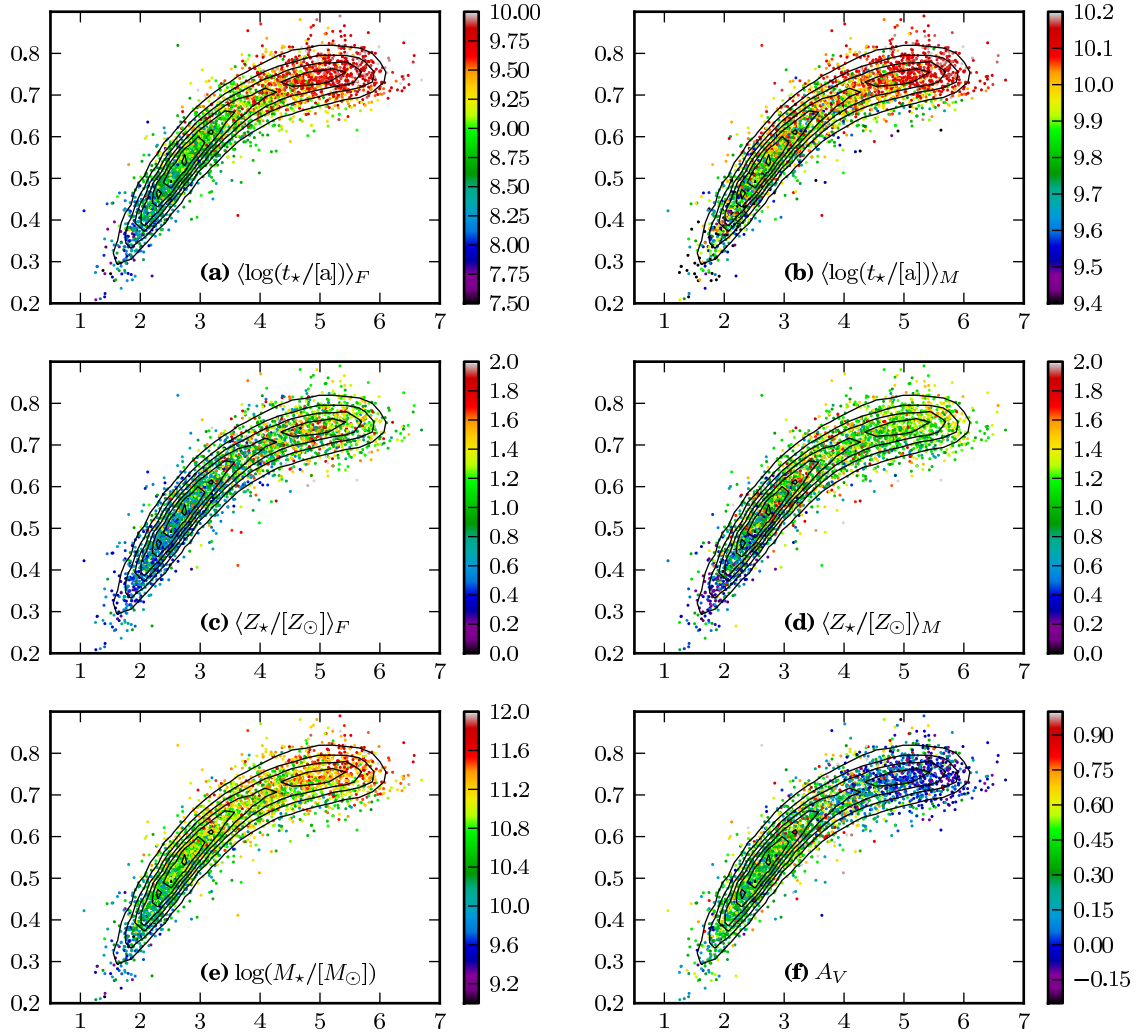
Figura 4.2: Propriedades físicas das galáxias em função de cor UV e cor óptica. O contorno das figuras representam os níveis referentes à figura 4.1, e os eixos horizontal e vertical são os mesmos utilizados naquela figura. As cores dos pontos nos painéis correspondem a: (a) Logaritmo da idade média das SSP componentes da galáxia, ponderada pelo fluxo. (b) O mesmo que a anterior, mas ponderada pela massa. (c) Metalicidade média das SSP componentes da galáxia, ponderada pelo fluxo. (d) O mesmo que a anterior, ponderada pela massa. (e) Logaritmo da massa estelar da galáxia, em massas solares. (f) Extinção por poeira na galáxia, na banda V.
