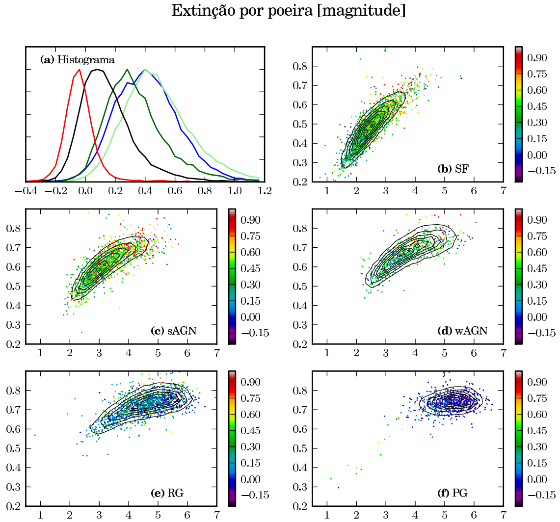
Figura 4.13: O mesmo que a figura 4.8, para a extinção por poeira na banda V das galáxias.
