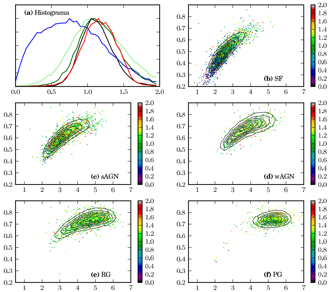
Figura 4.11: O mesmo que a figura 4.8, para a metalicidade estelar média das galáxias, ponderada pela massa.
