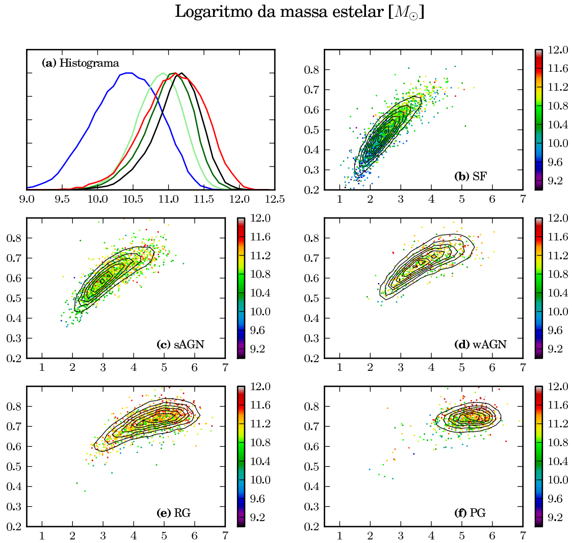
Figura 4.12: O mesmo que a figura 4.8, para o logaritmo da massa estelar das galáxias em massas solares.
