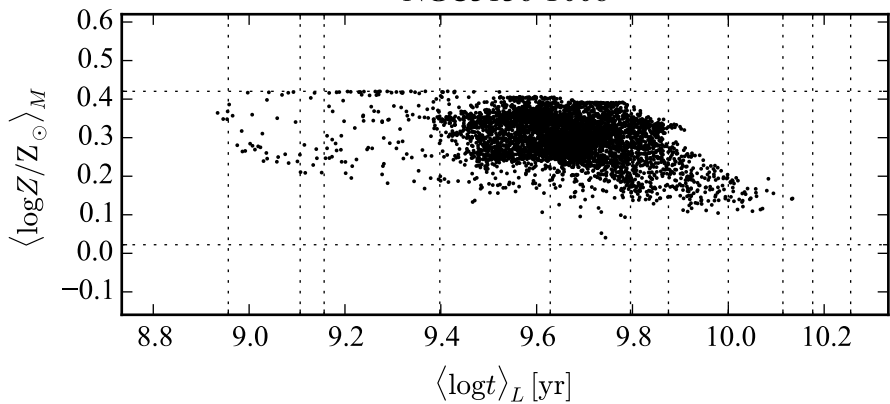
NGC3136 T008
