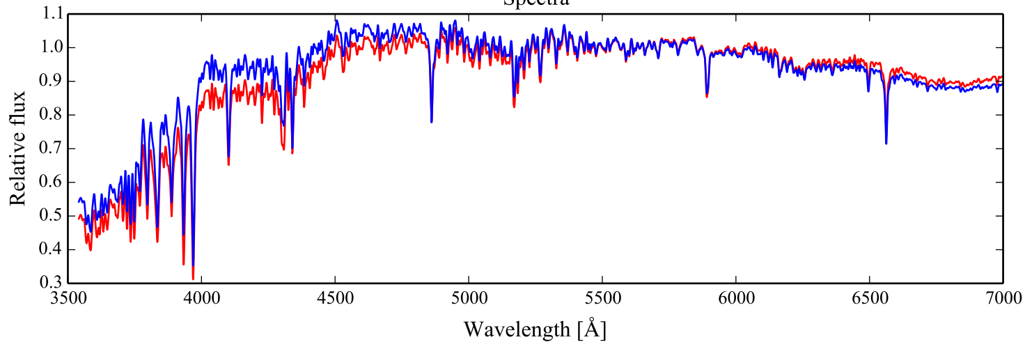
Spectra
