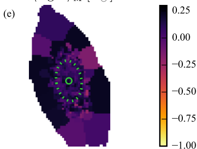
b^{\text{loc}}
