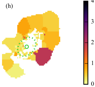
v_{\star} [\text{km s}^{-1}]
