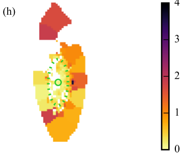
v_{\star} [\text{kms}^{-1}]
