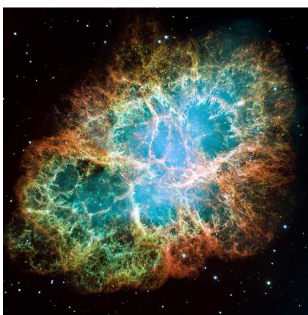
Το Νεφέλωμα του Καρκίνου. Είναι το υπόλειμμα μιας έκρηξης υπερκαινοφανούς (supernova), η οποία παρατηρήθηκε το 1054 μ.Χ. από Κινέζους αστρονόμους
