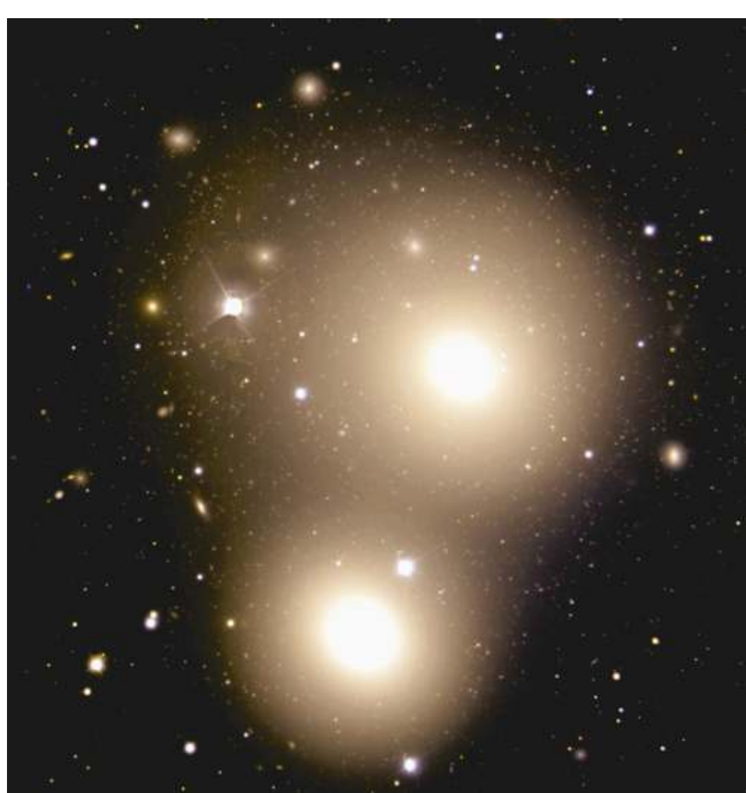
Dos galaxias elípticas: NGC 3311 y NGC 3309.
