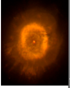
10 15 m: Nebulosa planetaria
