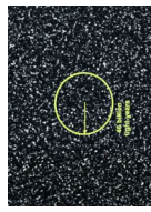
10 27 m: El Universo observable
