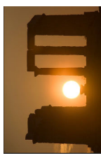
10 9 m: El Sol
