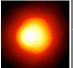
10 12 m: Supergigante roja
