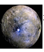
10 6 m: Planetas enanos
