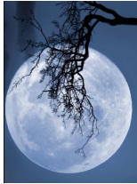
Las zonas de color gris de la Luna son derrames de lava endurecidos. Las zonas más claras son las más elevadas, ricas en calcio y aluminio.
