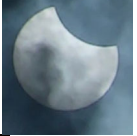
Cuando la Luna pasa delante del Sol se produce un eclipse de Sol. Aquí se muestra una foto de un eclipse parcial.
