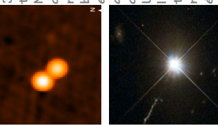
Deux galaxies, découvertes par le satellite IRAS dans l'infrarouge, vues par le télescope spatial Hubble dans le visible. Ces galaxies, 100 fois plus lumineuses dans l'infrarouge que dans le visible sont appelées ULIRGs (galaxies infrarouges ultralumineuses, en anglais). De nombreuses ULIRG montrent des signes d'interaction avec des galaxies voisines.
