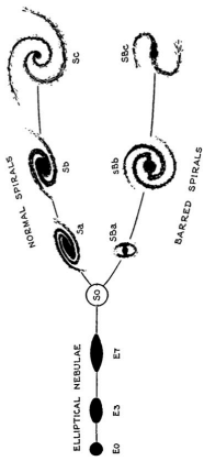
Il diagramma a diapason è stato ideato da Hubble nel suo libro del 1936 «The realm of the nebulae»
