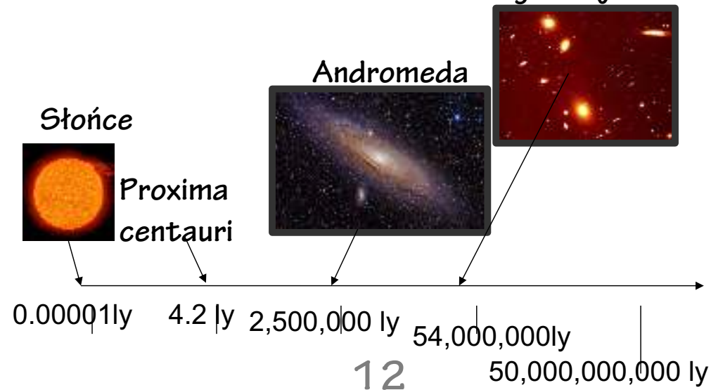
Gromada galaktyk Panna
