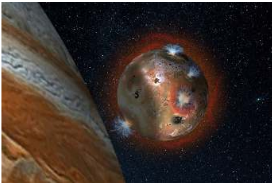
Artystyczne ujęcie Io z niektórymi wybuchającymi wulkanami. (SwRI/Andrew Blanchard/NASA)
