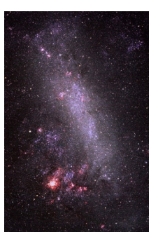
Norul Mare al lui Magellan, galaxia cea mai apropiată de Calea Lactee.
