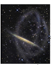
Fluxuri stelare slabe în jurul galaxiei spirale NGC 5907 văzută din lateral. Imagine de J. Gabany Blackbird Observatory.
