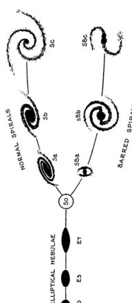
Diagrama diapazonului a fost desenată de Hubble în cartea sa din 1936 "Tărâmul Nebuloaselor"
