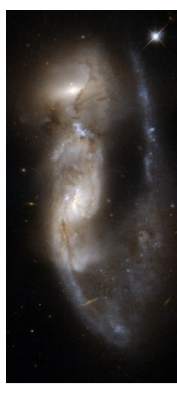
ESO 593-B: o pereche de galaxii care interacționează și care vor forma probabil o singură galaxie în viitor.
