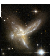
ESO 593-B: o pereche de galaxii care interacționează și care vor forma probabil o singură galaxie în viitor.
