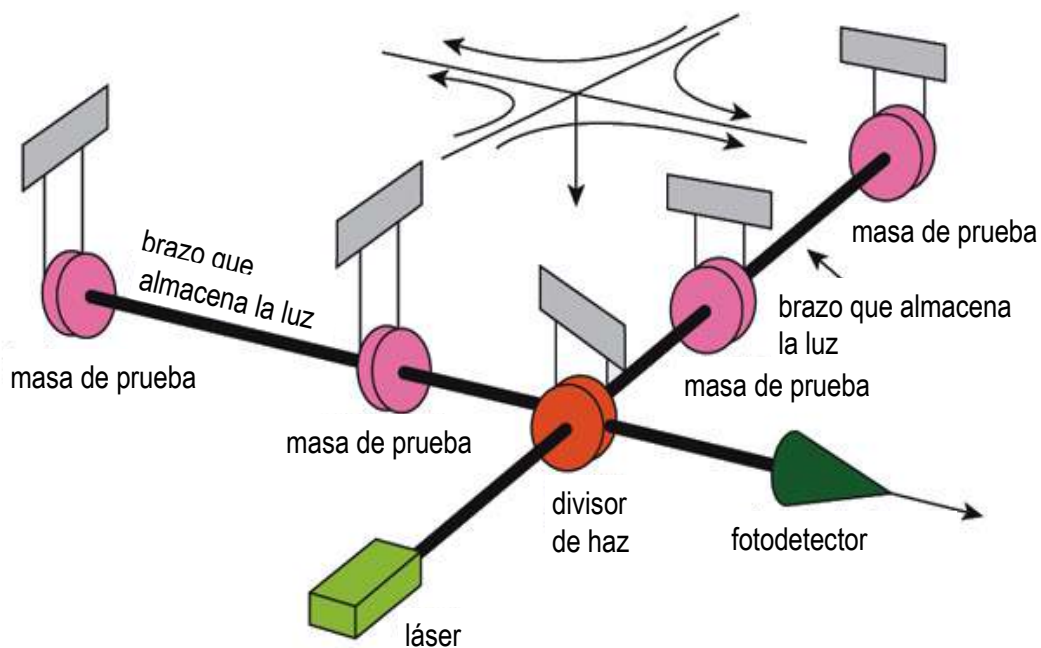
Esquema de funcionamiento de un detector interferométrico de ondas gravitacionales.
