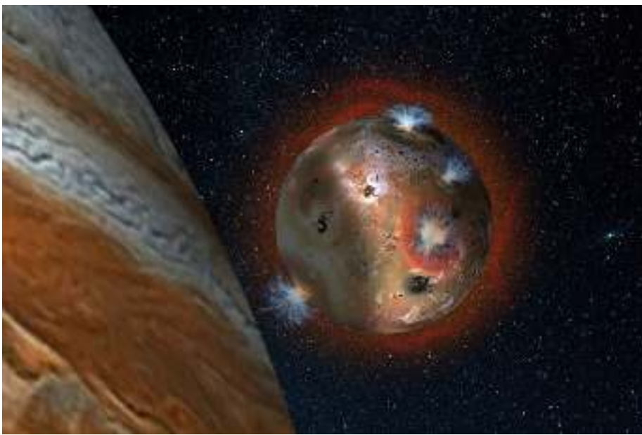
Vue d'artiste de Io, avec certains de ses volcans en éruption. (SwRI/Andrew Blanchard/NASA)
