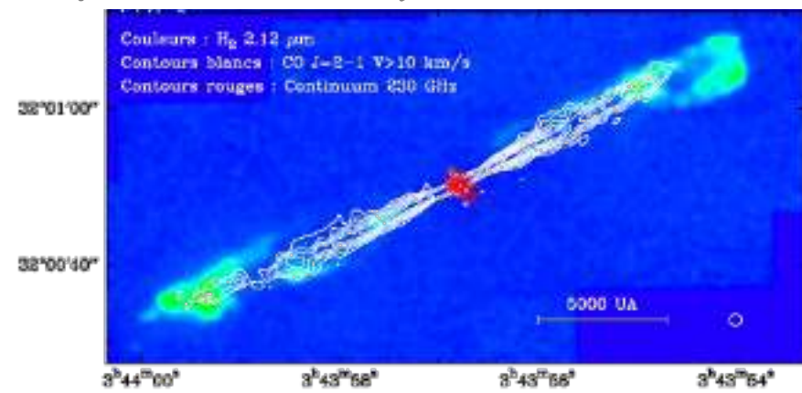
Émission radio de la molécule de CO (en blanc) dans les jets sortants d'une proto-étoile. Les contours rouges montrent l'émission radio de la poussière chaude, comme dans le système T Tauri (fausses couleurs),
