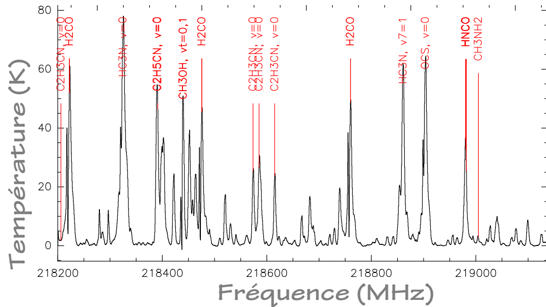
Raies d'émission de molécules dans la nébuleuse d'Orion. Chaque pic indique la présence d'une molécule (quelques exemples sont indiqués). Crédit L. Pagani.
