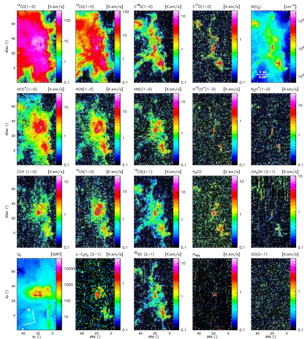
Une région de formation stellaire dans Orion tracée en ondes radio émises par différentes molécules (CO, HCO + , HCN, N 2 H + , C 2 H, CN, CS,... en fausses couleurs). Crédit P. Gratier et al. 2021.
