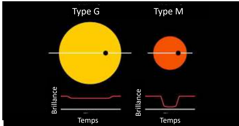
Variation de la brillance photométrique de deux étoiles lors d'une éclipse planétaire ( https://astro.unl.edu/ ).
