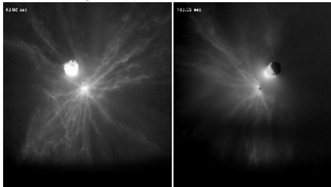
Obrazy wykonane przez nanosatelitę LICIACube na krótko po uderzeniu statku kosmicznego DART w księżyc Dimorphos. Uderzenie zmieniło orbitę księżyca, a także spowodowało powstanie chmury pyłu i głazów wokół księżyca i asteroidy.
