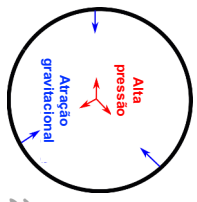
Uma estrela está em equilíbrio entre a ação da pressão térmica para fora e a ação da gravidade para dentro.
