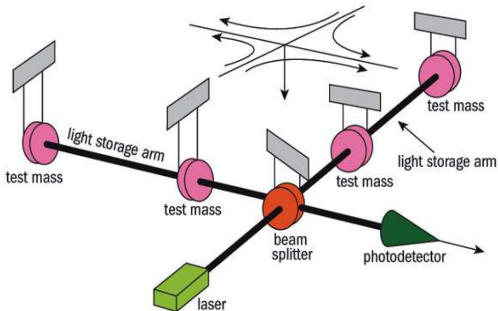
Diagrama operacional de um interferômetro detector de ondas gravitacionais.
