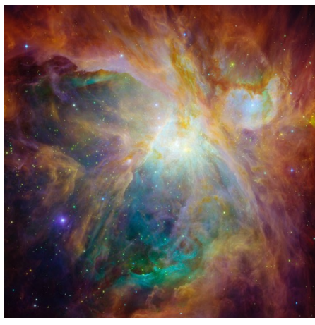
猎户座星云。这是天空中最明亮的星云，可以用肉眼看到。
