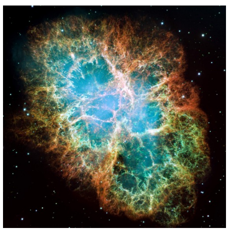
蟹状星云。这是一次超新星爆发留下的遗迹，这次爆发曾在 1054 年被中国天文学家记录下来。
