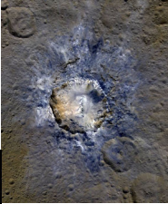
左图：谷神星是主小行星带中最大的小行星，也是一颗矮行星。图片展示了它表面那些神秘莫测的亮斑。
