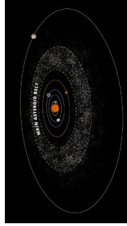
左图：位于火星与木星之间的主小行星带。
