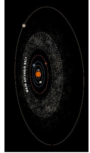
左图：位于火星与木星之间的主小行星带。
